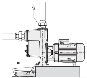
Fig. 3 Scarico Draining Entleerung Vidange Vaciado Avtappning Aftappen Αποστράγγιση Слив 排泵
