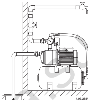
Fig. 2 Funzionamento in aspirazione Suction lift operation Saugbetrieb Fonctionnement en aspiration Funcionamiento en aspiración Sugande funktion Zugsituatie Θέση λειτουργίας με κάθστη αναρρόφηση Работа выше уровня жидкости 负吸水头工作
