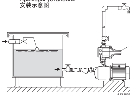
Fig. 1 Funzionamento sotto battente Positive suction head operation Zulaufbetrieb Fonctionnement en charge Funcionamiento bajo carga Tillrinning sugsidan Töölöpsuutite Θέση λειτουργίας με θετική αναρρόφηση Работа под гидравлическим напором 正压上水头的操作
