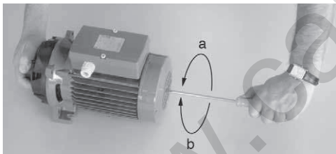
Fig. 3 Smontaggio (a) e rimontaggio (b) girante
