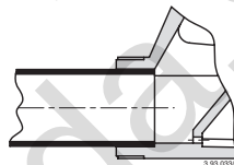
Рис. 1 Соединение приклеиванием.
