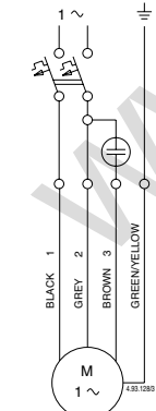
Схема подключения с монофазными двигателями
