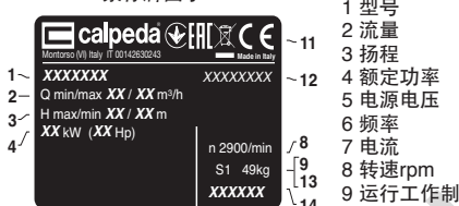
电机标牌图示
