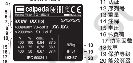
电机标牌图示
