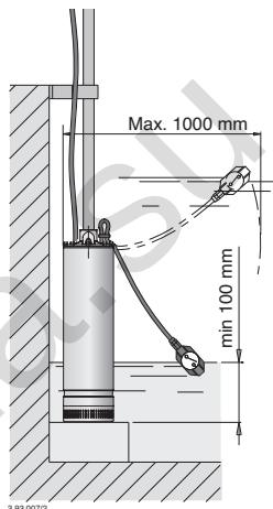
Pomp met vlotterschakelaar
