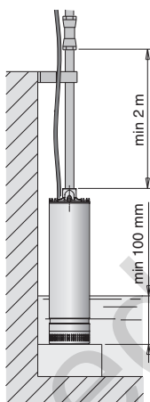
Модификация без поплавкового выключателя
