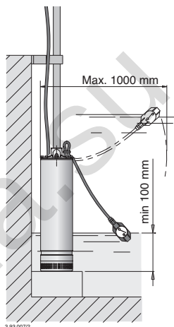
Exécution avec interrupteur à flotteur
