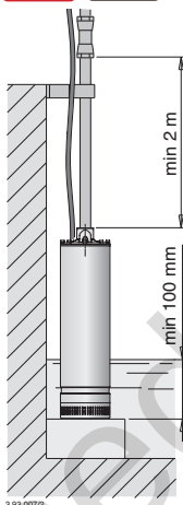
Konstruktion utan nivåbrytare
