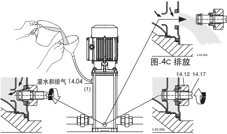
图.4a 灌水: 内部通道打开 图.4b 运行: 内部通道关闭
