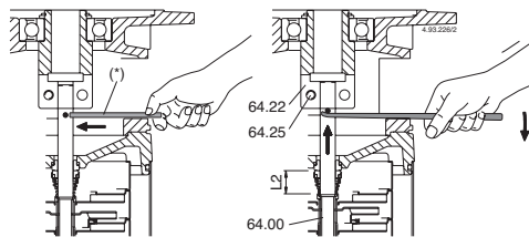
Σχ.6α Σταθεροποίηση ρότορα με απασφαλισμένο άξονα στην σύζευξη. Σχ.6β Ανύψωση ρότορα για ασφαλισμένο άξονα στην σύζευξη.
