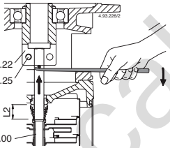
图.6b 转子提升,把轴固定在联轴器的位置。
