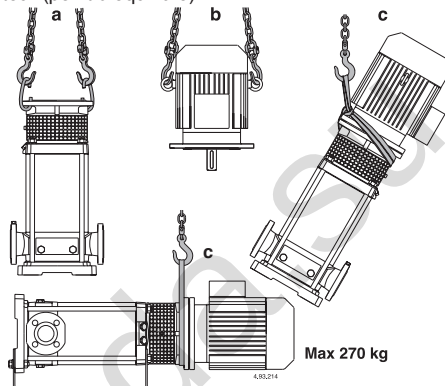
Fig. 1 a b c ILevage de la pompe sans moteur ILevage du moteur seul ILevage de la pompe avec moteur
