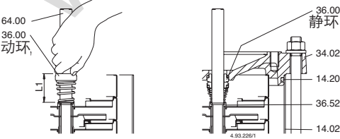
图5 插入机械密封
