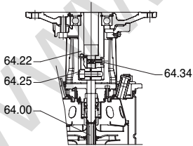
图.6a 转子静止,和轴一起均未被联轴器锁住 (*)提升用的销
