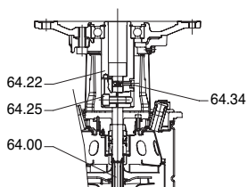
Σχ.6α Σταθεροποίηση ρότορα με απασφαλισμένο άξονα στην σύζευξη. Σχ.6β Ανύψωση ρότορα για ασφαλισμένο άξονα στην σύζευξη.
